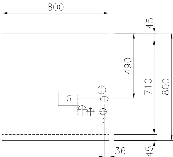
Boven aanzicht
